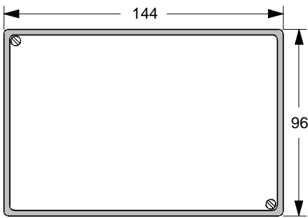
Vorderansicht; Aufbauregler
