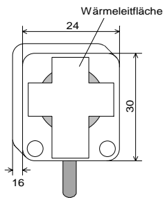
Anlegefühler Typ 3111
