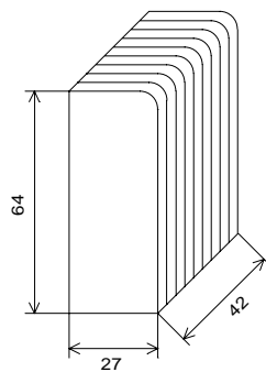
Witterungsfühler Typ 3115
