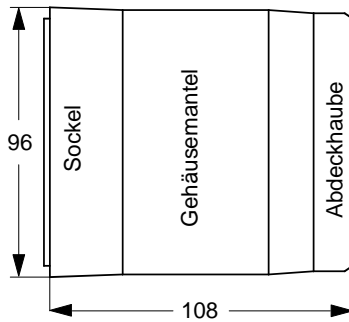
Seitenansicht; Aufbauregler
