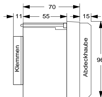
Seitenansicht; Einbauregler
