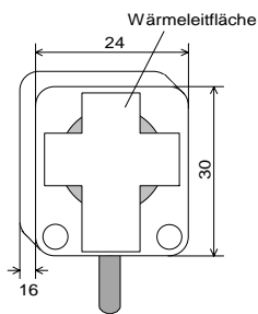
Anlegefühler Typ 3111
