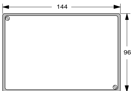
Vorderansicht; Aufbauregler
