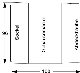
Seitenansicht; Aufbauregler
